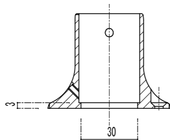
A-A断面図
